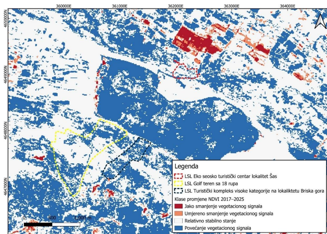
Slika 33. Prostorna raspodjela klasa promjene vegetacionog signala (NDVI), 2017–2025
